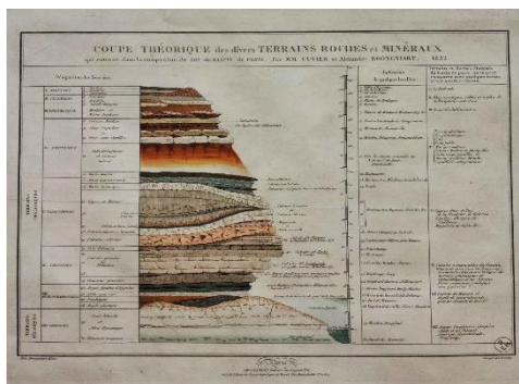
Coupe géologique 1832 (Cuvier et Brongniart)
